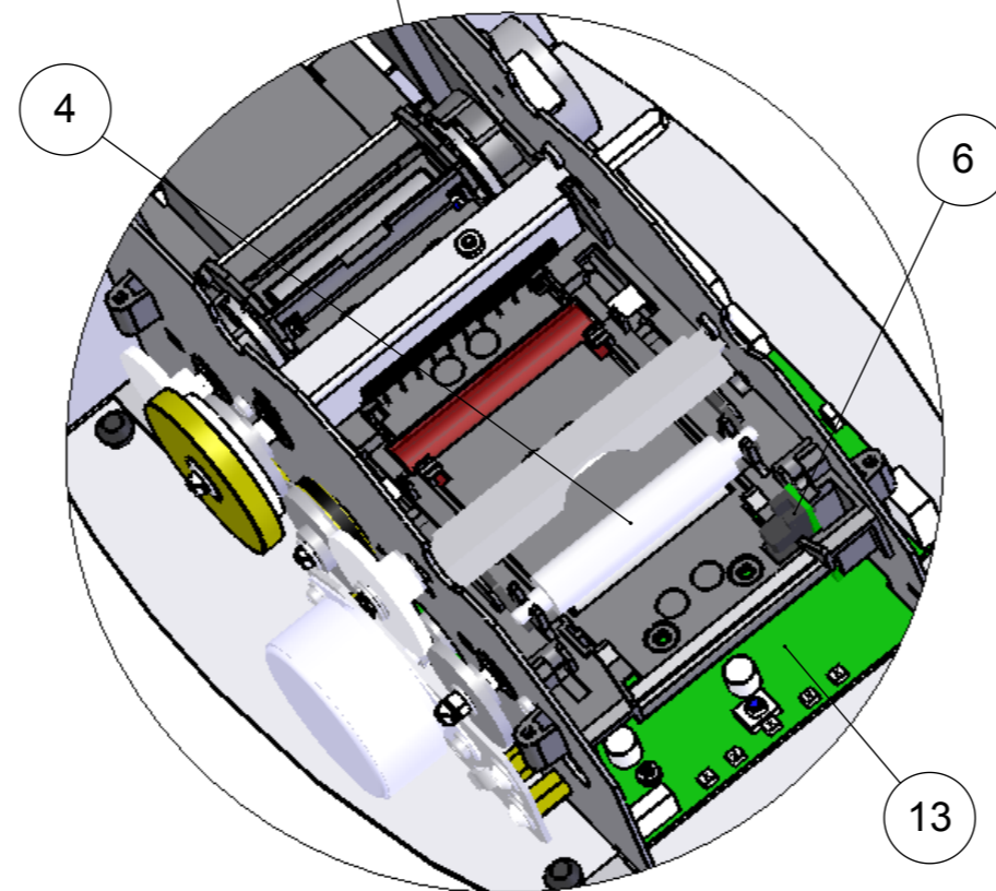
DÉTAIL A ECHELLE 1 : 2
